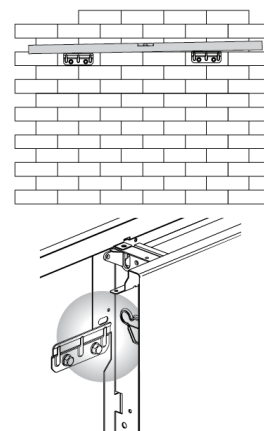
Montaggio a parete unità con mobiletto
