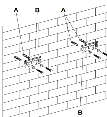
Montaggio a parete unità con mobiletto
