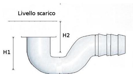
Scarico condensa laterale
